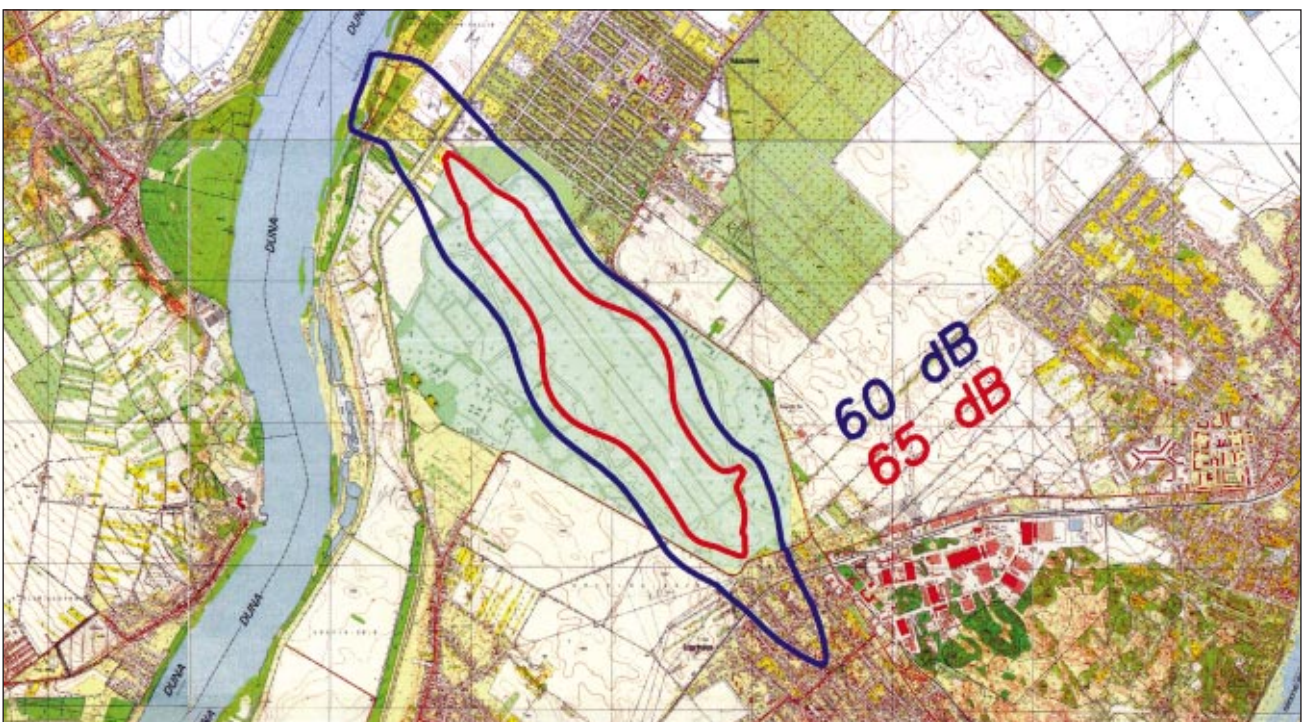
A tököli repülőtér és a számított ISOPHON görbék
